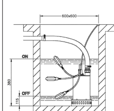
FIG. 4 BEST 2-3-4-5 MA
